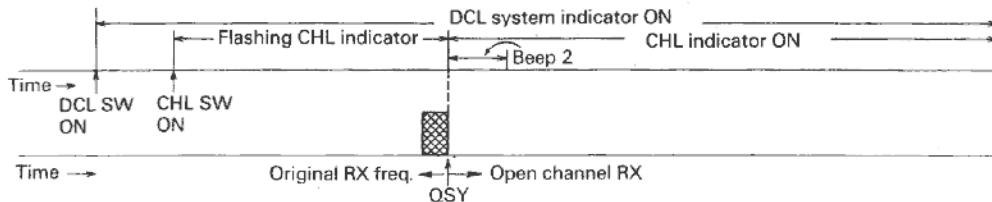
Fig. a. Simplex mode
